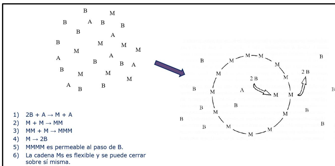
FIGURA 2. Modelo computacional autopoiético, inspirado en reacciones químicas de síntesis y lisis (Maturana y Varela, 1998: 22)
